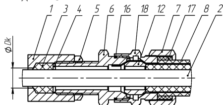
ж) монтаж бронированным кабелем в кабельном вводе KBY
