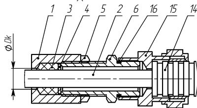
г) монтаж кабелем в металлорукаве в кабельном вводе KBM
