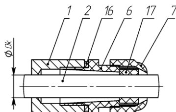
е) монтаж в кабельном вводе KBП12
