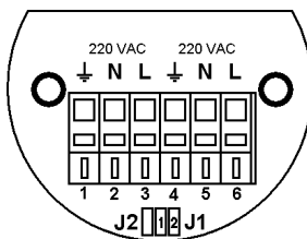
б) BC-07е-О-3(И)-230VAC
