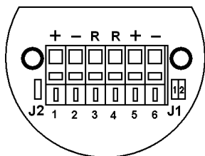
а) BC-07е-О-3(И)-24VDC
