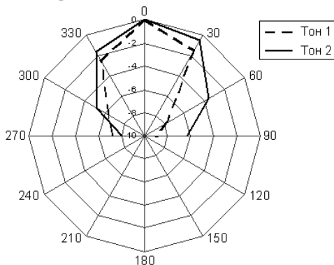
Рисунок 8. Диаграмма направленности звука BC-07е-О-3(И).
