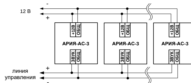
Рис.1. Схема подключения.
