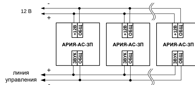
Рис.1. Схема подключения.
