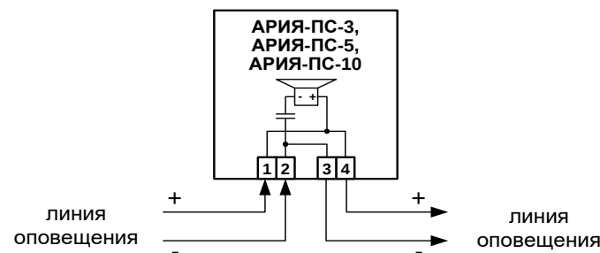
Рис.1. Схема подключения.
