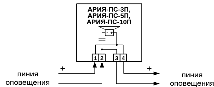
Рис.1. Схема подключения.
