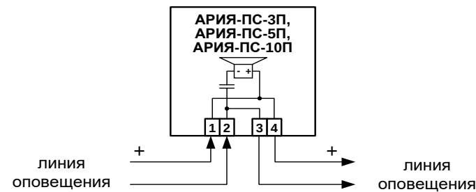
Рис.1. Схема подключения.
