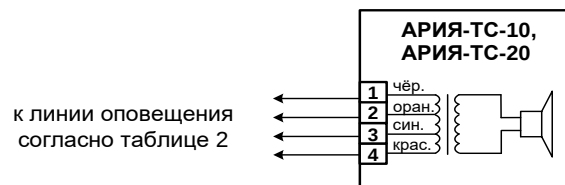
Рис.1. Схема подключения.
