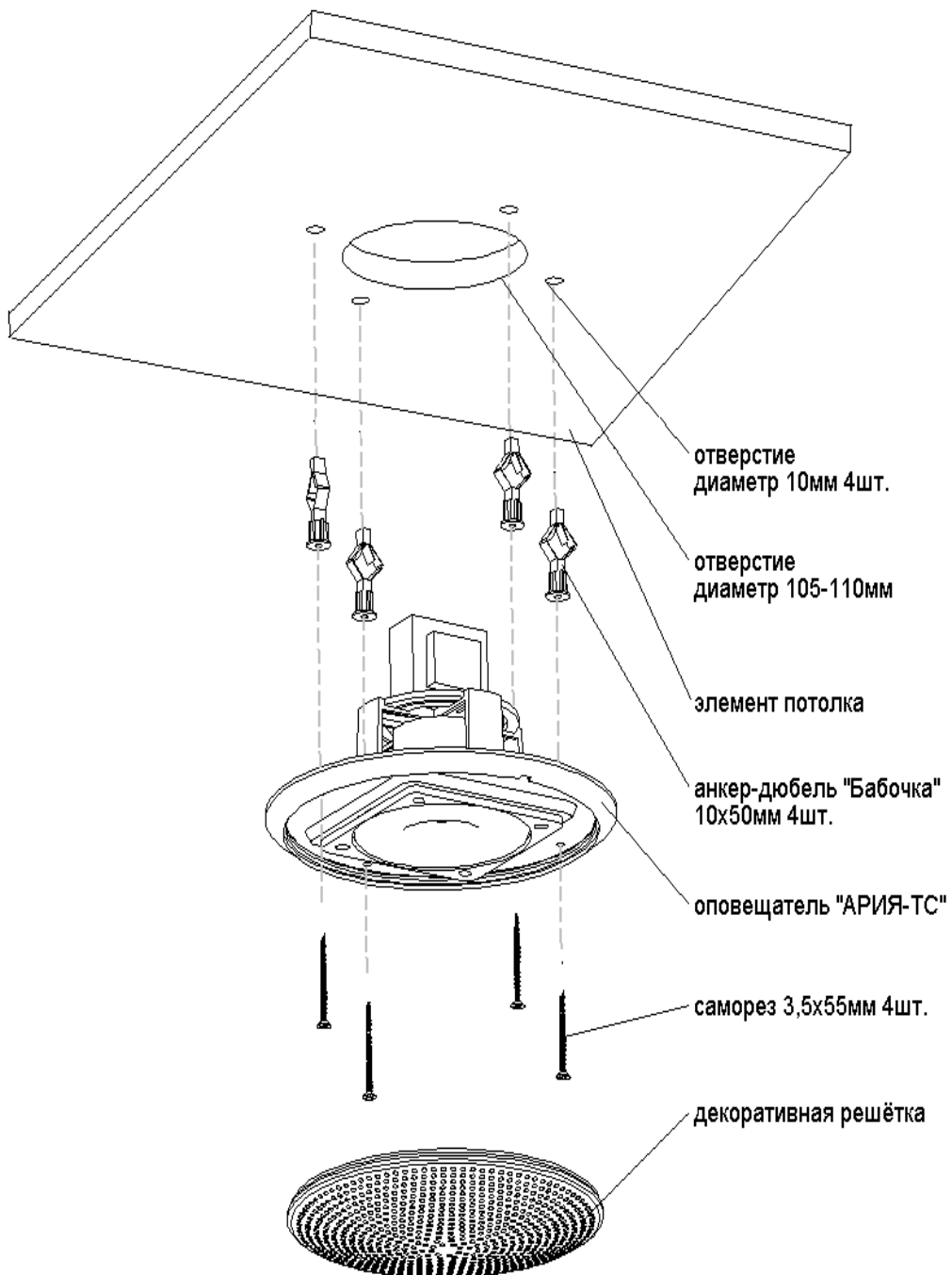
Рис.2. Монтажная схема.
