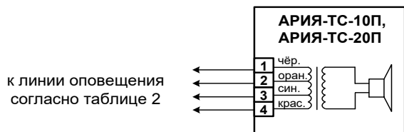
Рис.1. Схема подключения.
