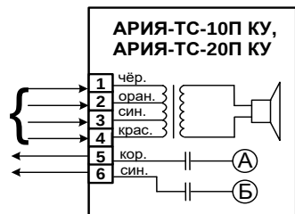
Рис.1. Схема подключения.
