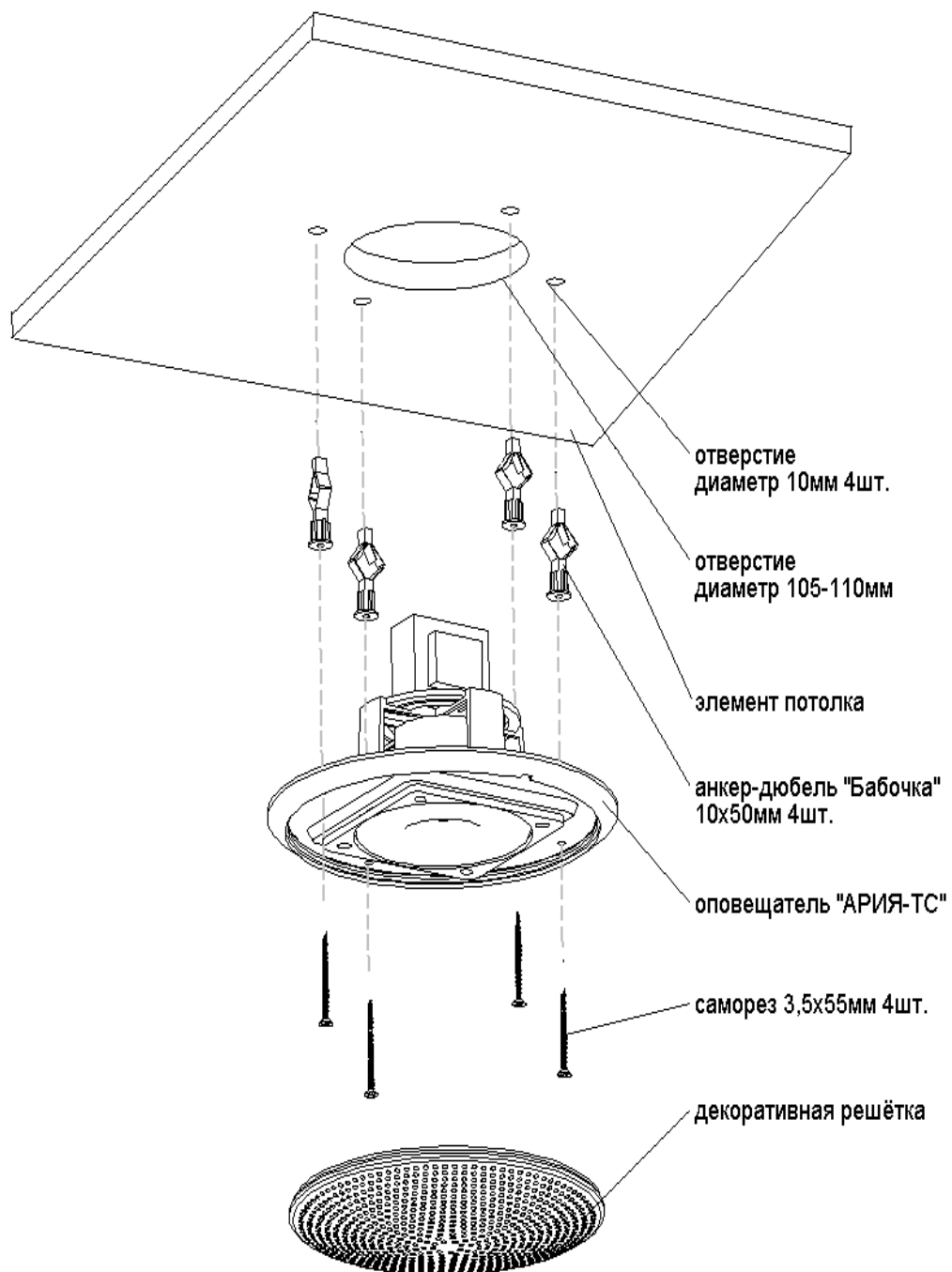
Рис.2. Монтажная схема.
