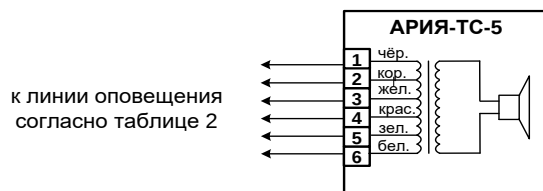
Рис.1. Схема подключения.
