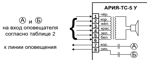
Рис.1. Схема подключения.
