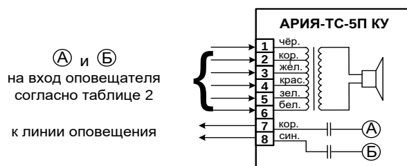
Рис.1. Схема подключения.
