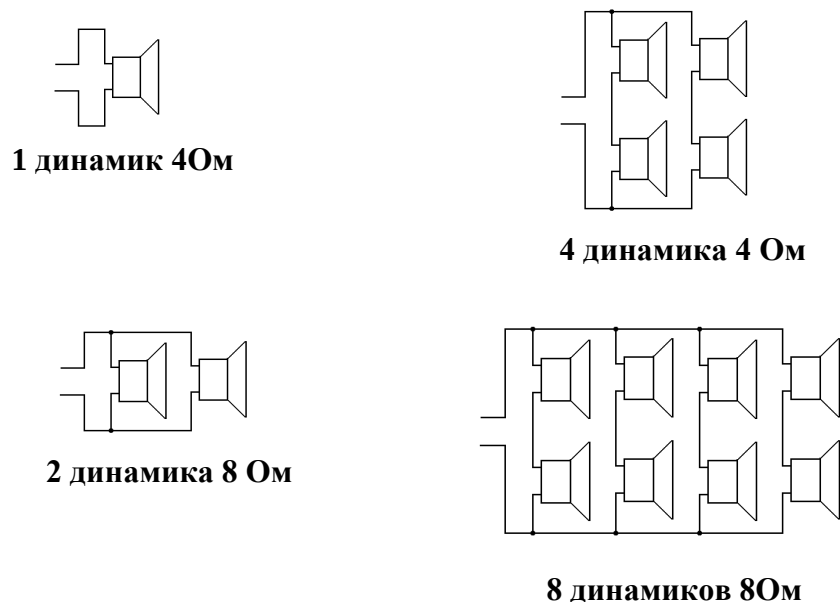
Рис.2 Типовые схемы подключения акустических систем АС-У-5
