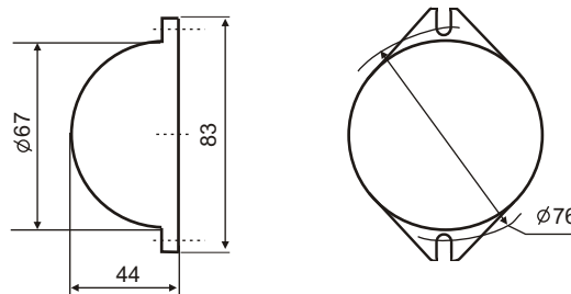
Рис.1. Габаритные и установочные размеры
