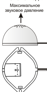
Рис.2 Схема подключения и диаграмма направленности оповещателя .
