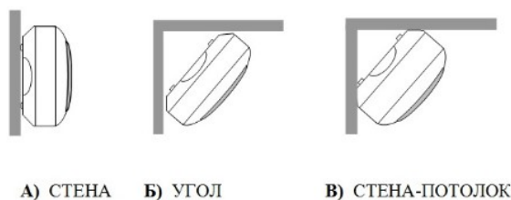
Рис.2 Варианты установки оповещателя
