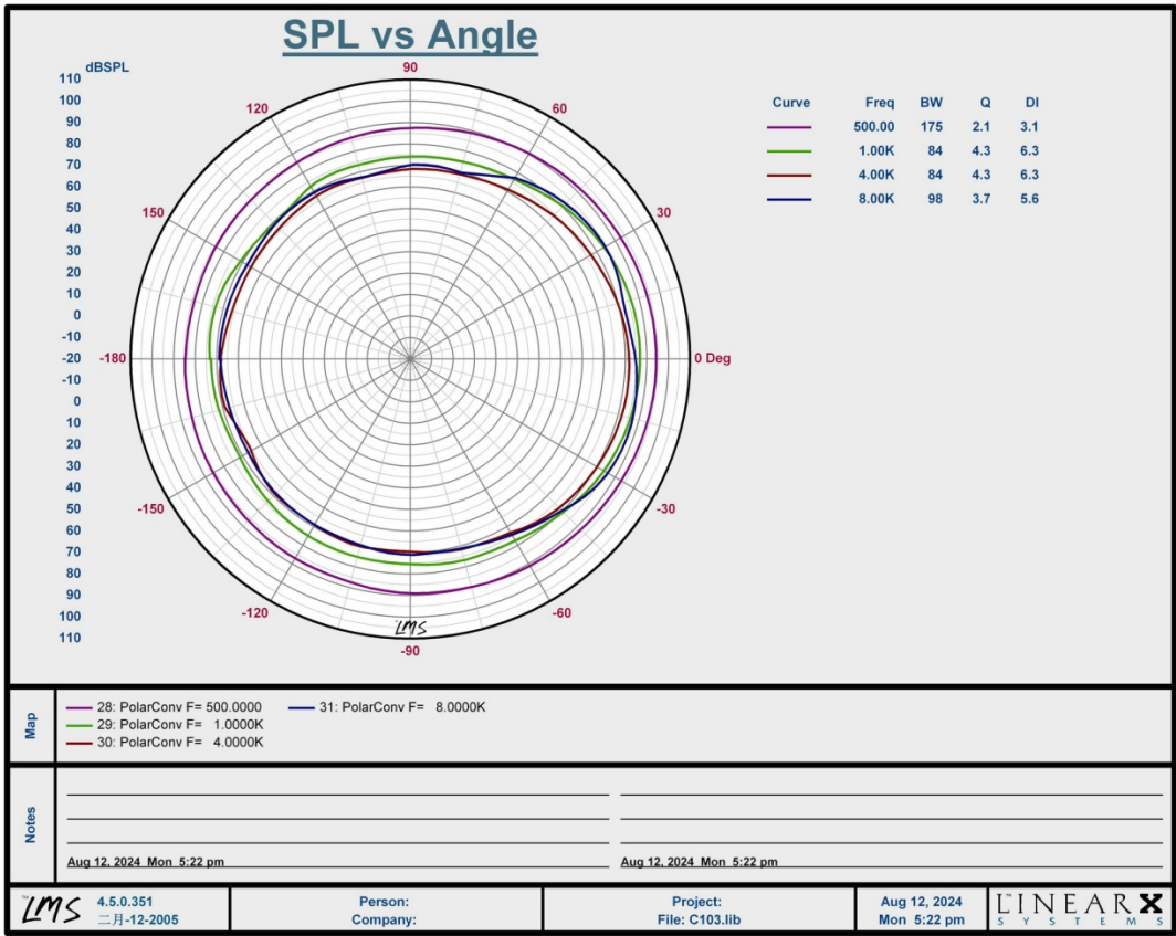
Диаграмма направленности
