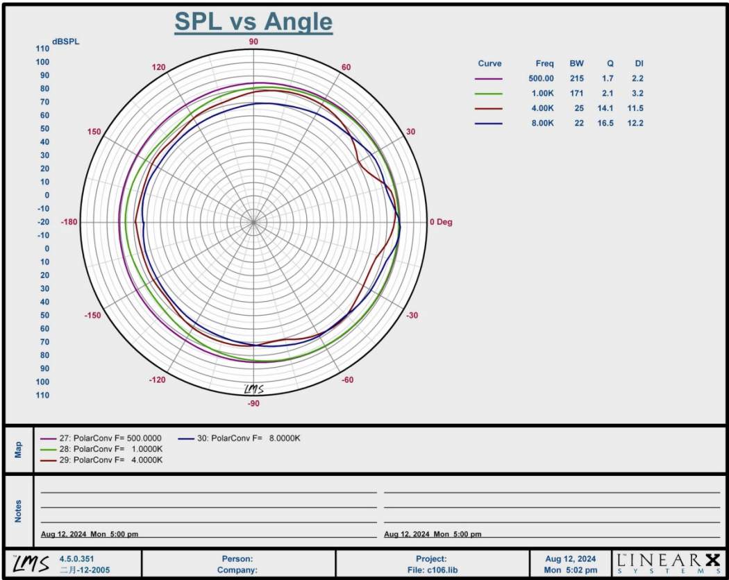
Диаграмма направленности
