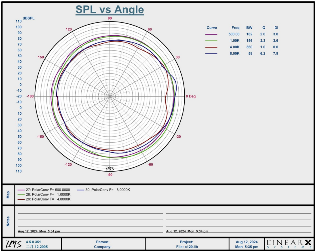
Диаграмма направленности
