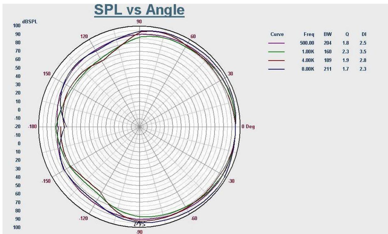
Диаграмма направленности
