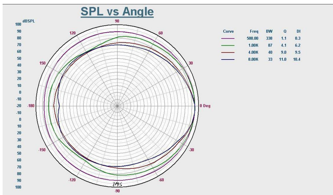
Диаграмма направленности
