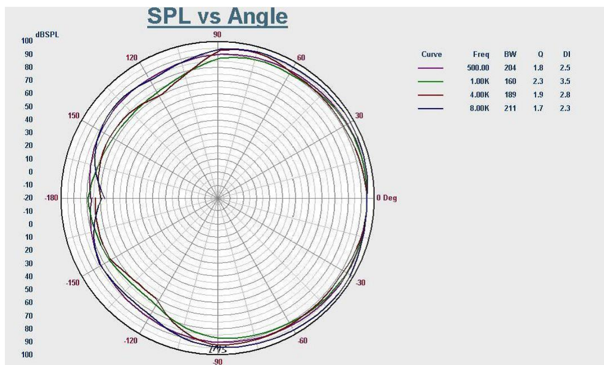
Диаграмма направленности
