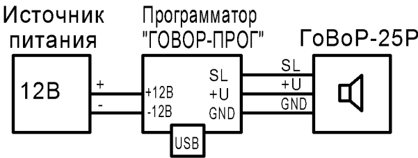
Рис. Б.5 Схема подключения GoBoP-25P к программатору GoBoP-ПРОГ при загрузке сообщений.
