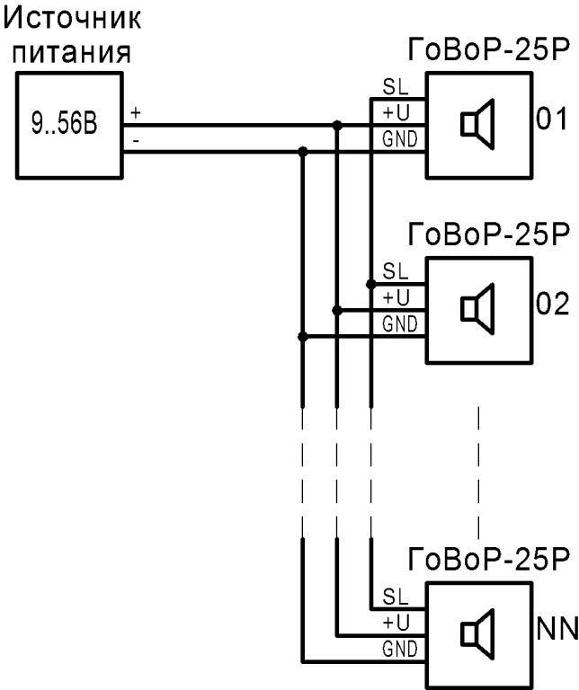
Рис. Б.4 Схема подключения нескольких GoBoP-25P с синхронизацией.
