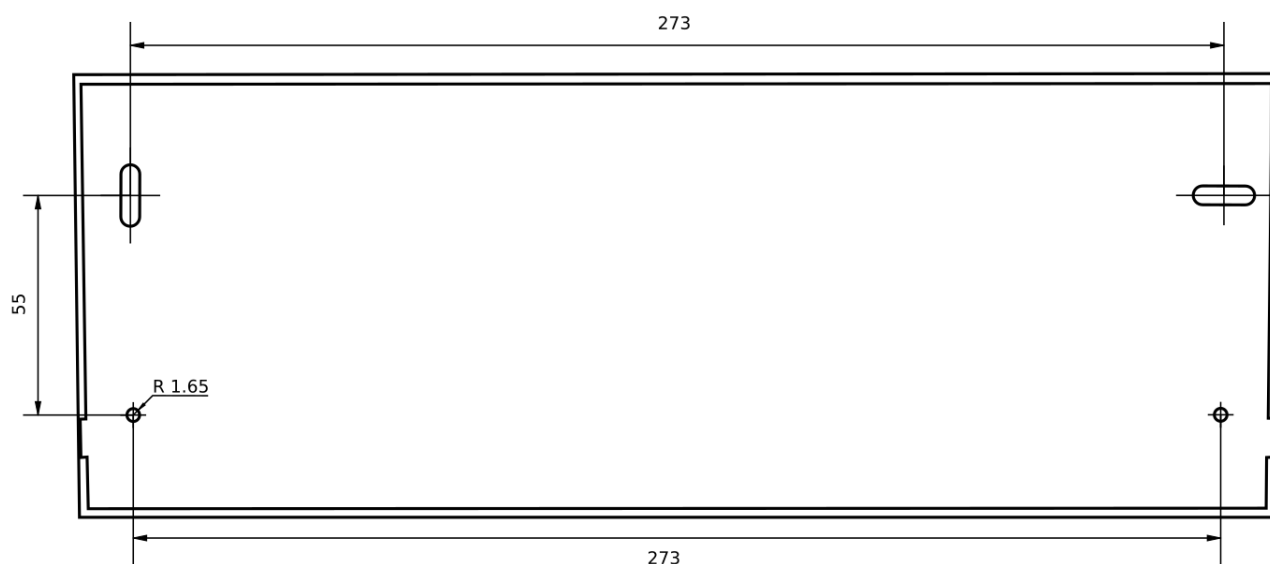
Рисунок 2.4 Монтажные размеры
