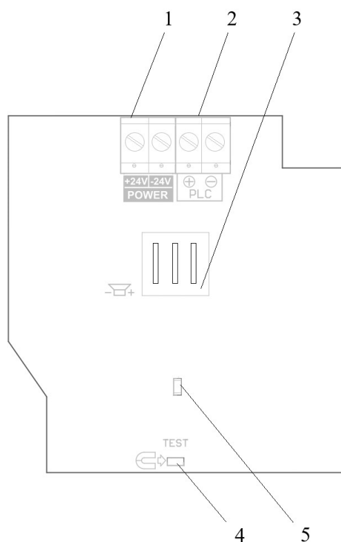
Рисунок 2 - Внутреннее устройство оповещателя
