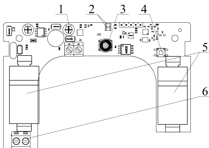
Рисунок 2 - Внутреннее устройство оповещателя
