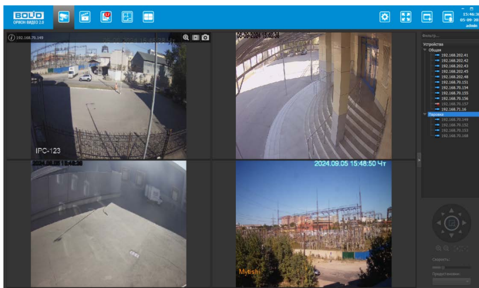
Рисунок 7.37 – Живое видео
