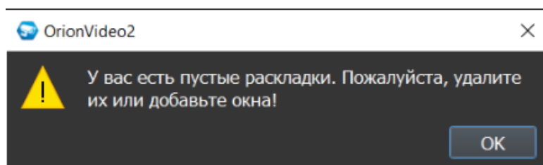
Рисунок 7.52 – Окно сообщения
