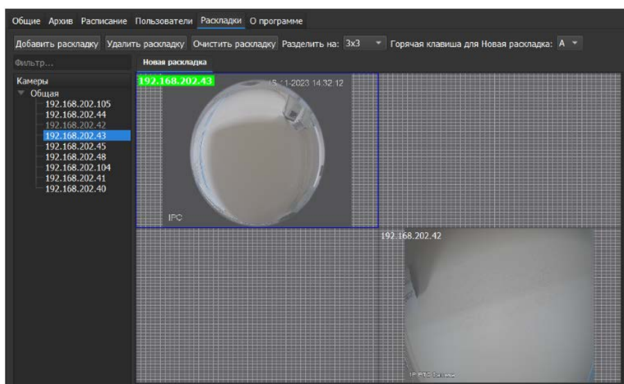
Рисунок 7.51 – Создание раскладки
