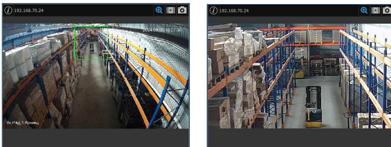
Рисунок 7.34 – Цифровой зум
