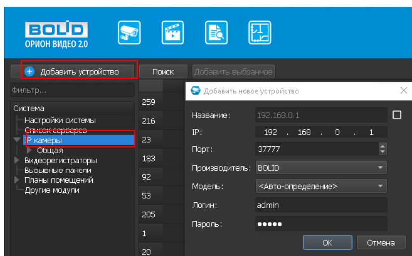
Рисунок 6.6 – добавление видеокамеры
