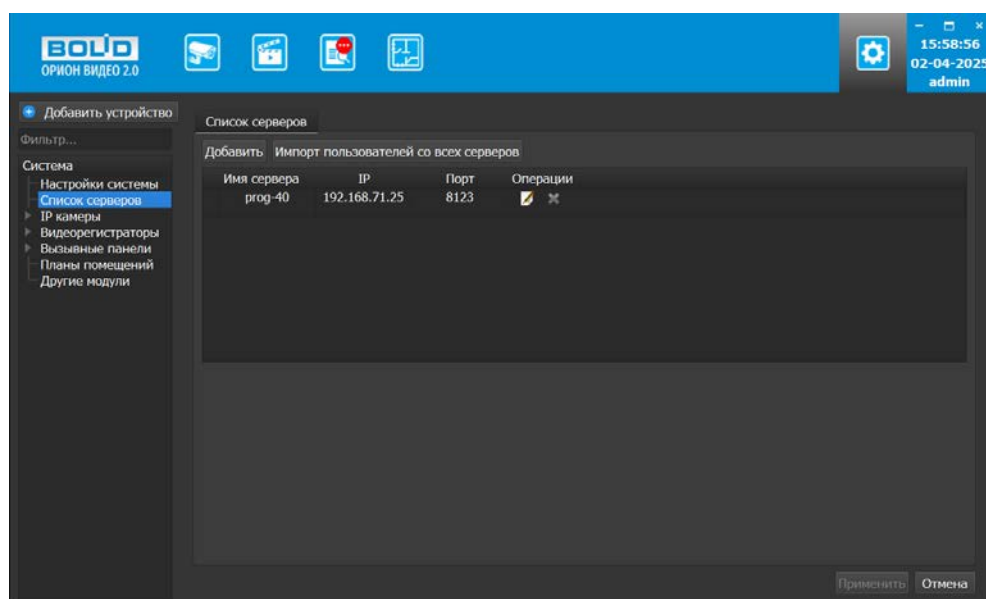
Рисунок 4.30 – Список серверов
