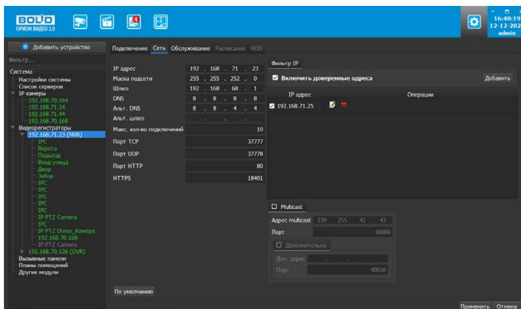
Рисунок 6.51 – Фильтр IP
