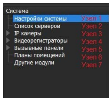
Рисунок 5.1 – Дерево системы
