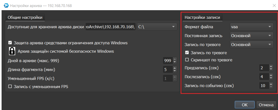
Рисунок 8.10 – Настройки записи
