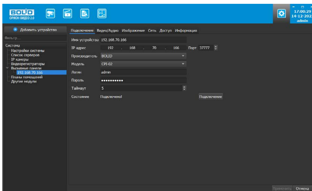
Рисунок 6.69 – Вкладка «Подключение»
