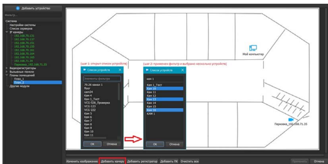
Рисунок 10.8 – Добавление устройств
