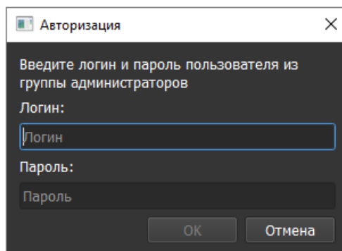
Рисунок 2.27 – Форма авторизации
