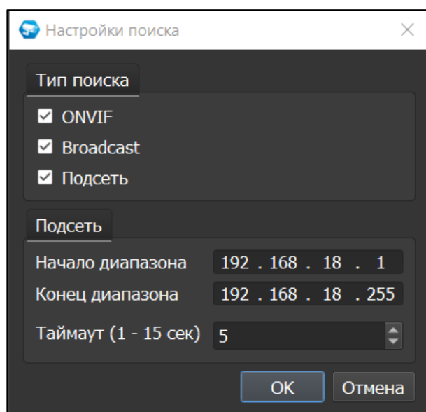
Рисунок 6.44 – Настройки поиска
