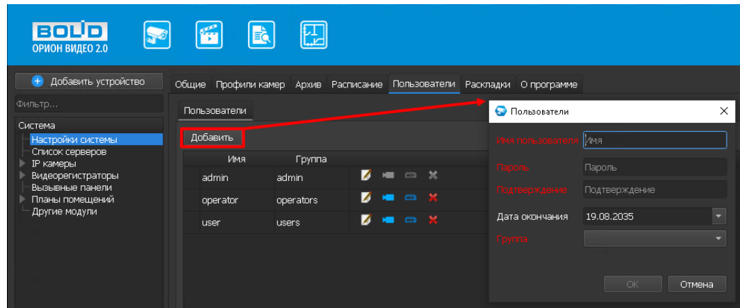
Рисунок 5.4 – Добавление пользователя
