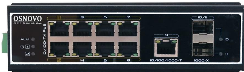
Рис.1 Коммутатор SW-60812/I (вид спереди)
