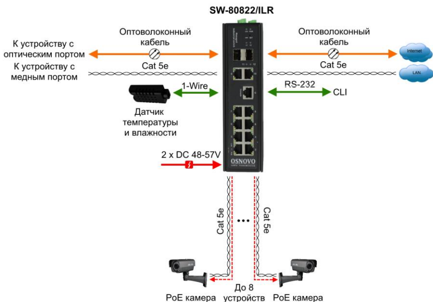
Рис. 5 Типовая схема подключения коммутатора SW-80822/ILR
