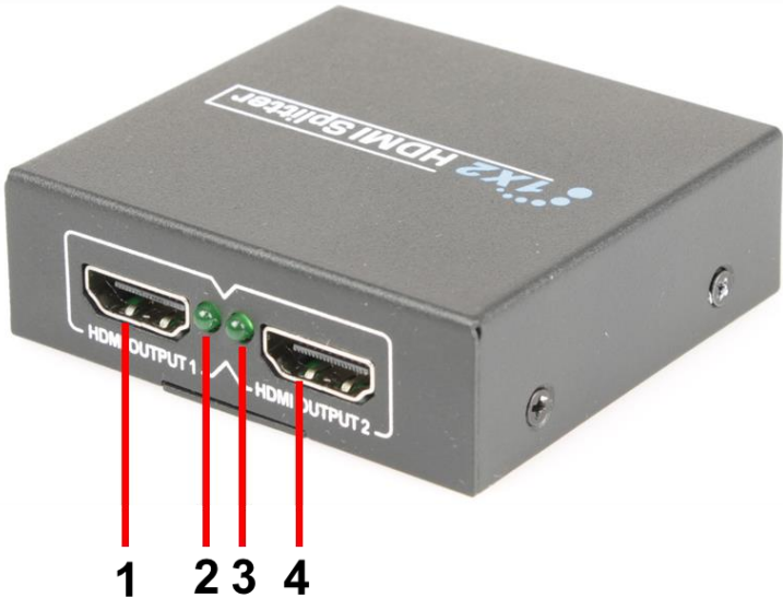
Рис.3 HDMI разветвитель D-Hi1021, разъемы и индикаторы на задней панели
