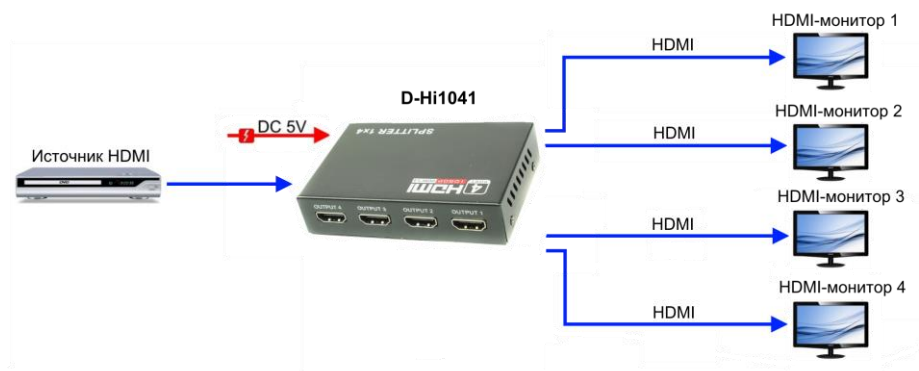
Рис.4 Типовая схема подключения HDMI разветвителя D-Hi1041
