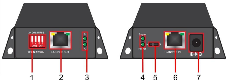
Рис.3 Панели подключения удлинителя E-PoE/1A
