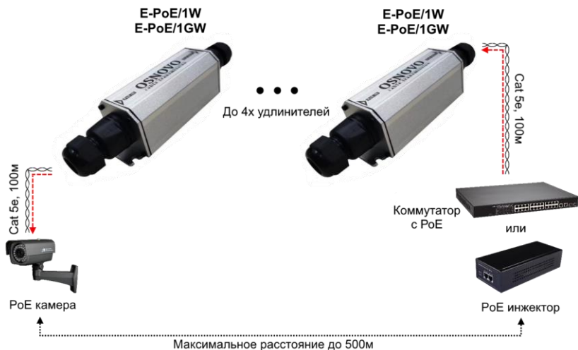
Рис.3 Схема подключения удлинителей E-PoE/1W, E-PoE/1GW.
