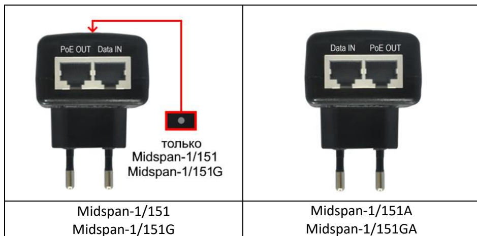
Рис.1 Разъемы подключения
