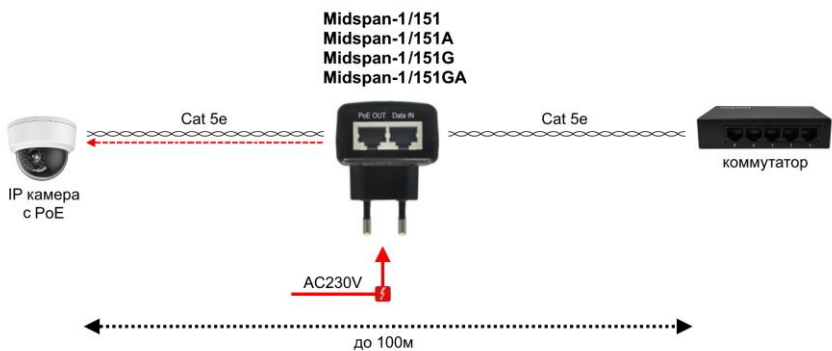
Рис.2 Схема подключения
