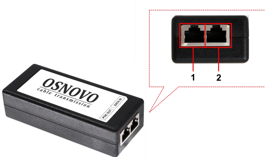
Рис. 2 Midspan-1/300G, Midspan-1/300GA, разъемы передней панели
