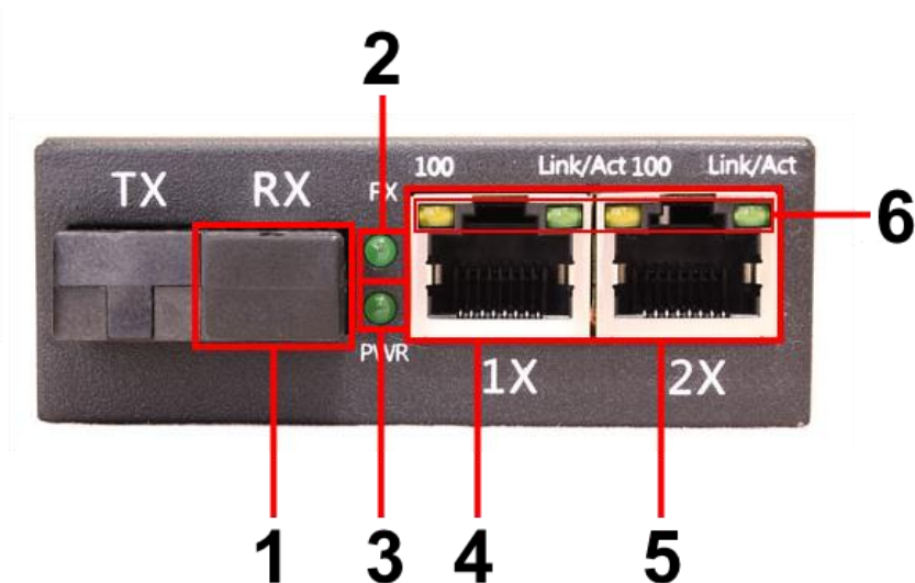
Рис. 4 Медиаконвертер ОМС-100-21S5b, разъемы и индикаторы на передней панели
