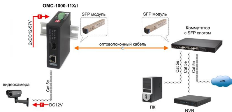
Рис.4 Типовая схема подключения медиаконвертера ОМС-1000-11Х/І
