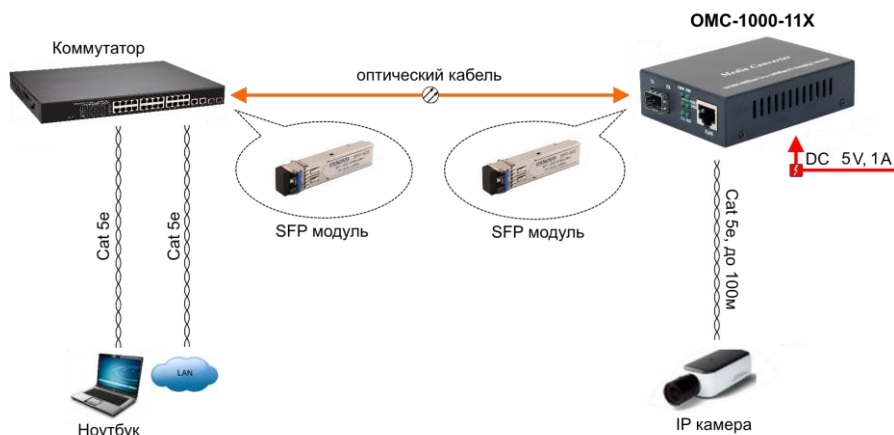
Рис.5 Типовая схема подключения медиаконвертера ОМС-1000-11Х
