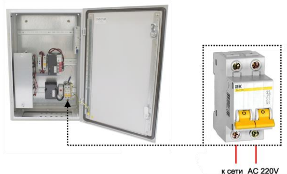
Рис.4 Точка подключения уличной станции к сети 220V переменного тока на примере модели OS-46TB1
