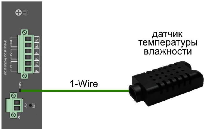
Рис.6 Схема подключения внешнего датчика температуры и влажности
