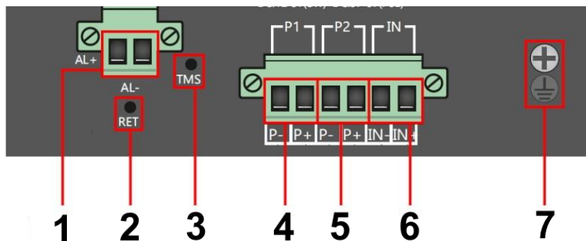
Рис. 3 Коммутатор SW-81602/ILS(port 90W, 600W), разъемы и кнопки на верхней панели
