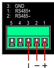
Рис.10 Клеммные колодки для подключения устройств с интерфейсами RS485 к передатчикам / приемникам TA-Hxx-15F / RA-Hxx-15F
