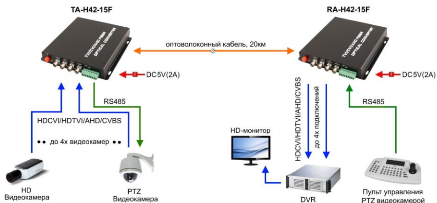
Рис.9 Типовая схема подключения передатчиков и приемников на примере TA-H42-15F и RA-H42-15F
