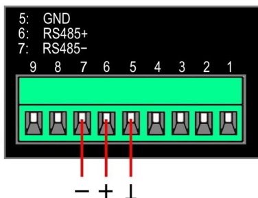
Рис.10 Клеммные колодки для подключения устройств с интерфейсами RS485 к передатчикам / приемникам TA-Hxx-15F / RA-Hxx-15F
