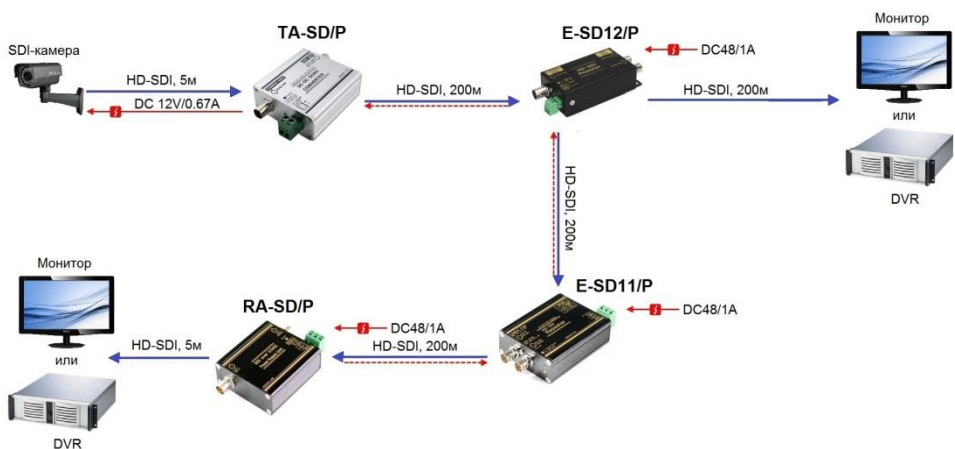
Рис. 9 Схема подключения передатчика TA-SD/P, повторитель-разветвителя E-SD12/P, , повторителя E-SD11/P и приёмника RA-SD/P.
