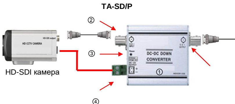
Рис.3 Элементы TA-SD/P.
