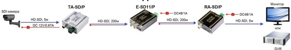
Рис.7 Схема подключения передатчика TA-SD/P, повторителя E-SD11/P и приёмника RA-SD/P.
