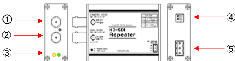
Рис. 5 Элементы E-SD11/P
