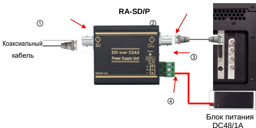
Рис.4 Элементы RA-SD/P.
