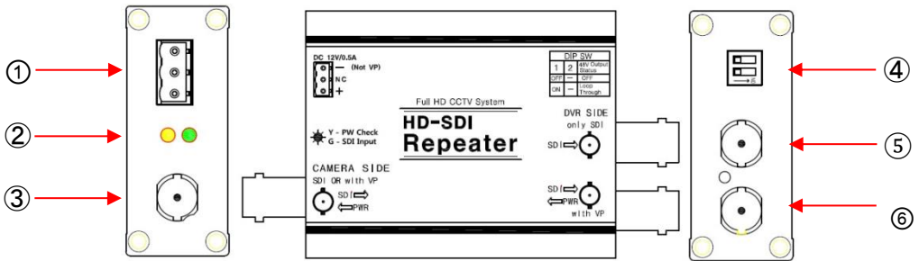
Рис. 6 Элементы E-SD12/P
