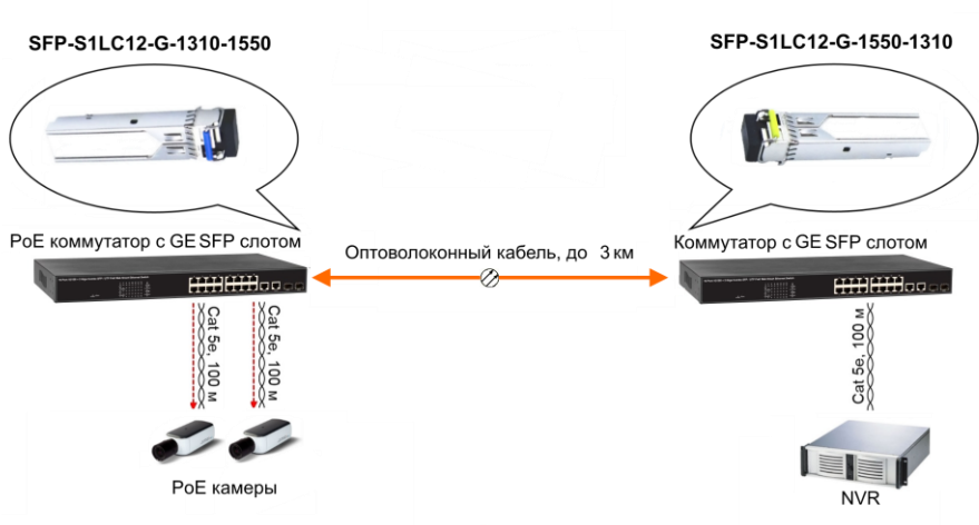
Рис.4 Типовая схема подключения SFP модулей SFP-S1LC12-G-1310-1550, SFP-S1LC12-G-1550-1310
