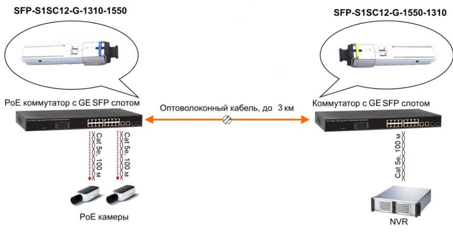
Рис.4 Типовая схема подключения SFP модулей SFP-S1SC12-G-1310-1550, SFP-S1SC12-G-1550-1310
