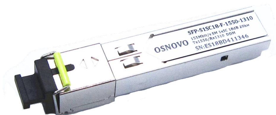
Рис.1 SFP модули, внешний вид на примере SFP-S1SC18-F-1310-1550, SFP-S1SC18-F-1550-1310 (модули с промышленным исполнением выглядят аналогично)
