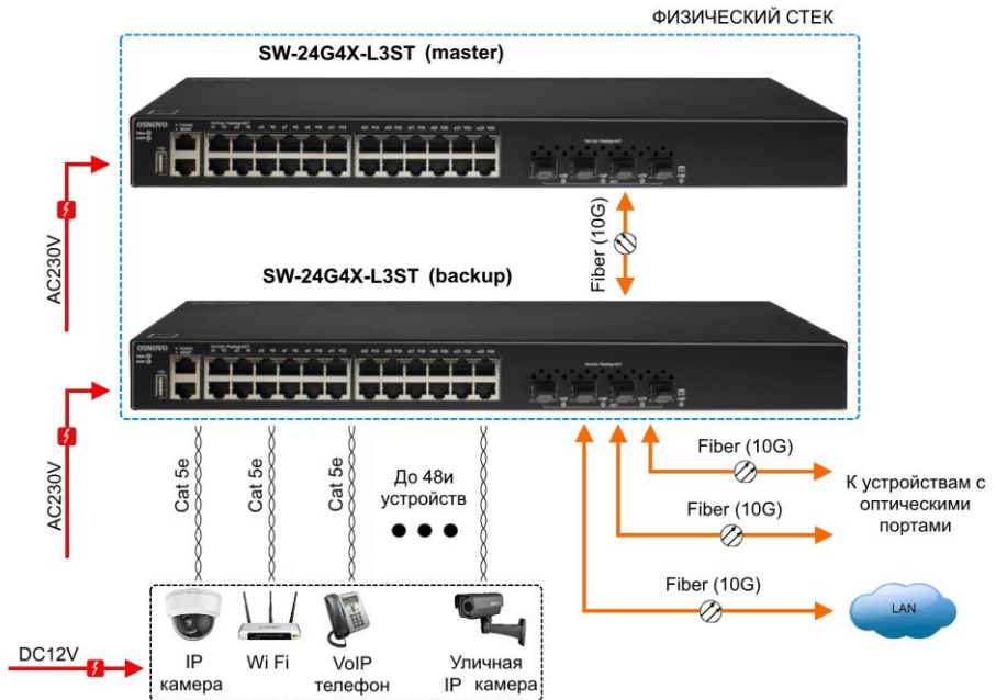
Рис.8 Стечное подключение коммутаторов на примере SW-24G4X-L3ST.
