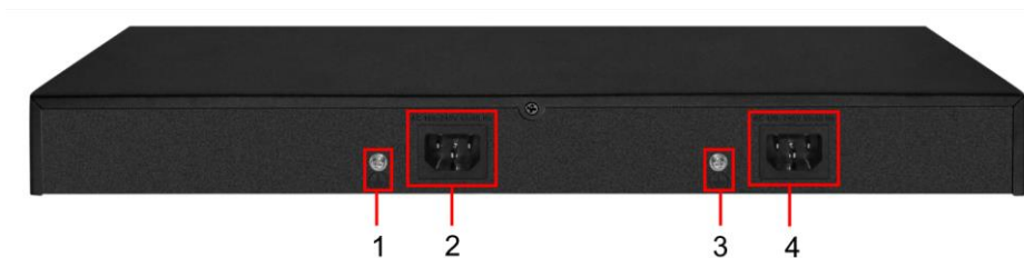
Рис.3 Коммутатор SW-32G4X-1L, разъемы на задней панели.
